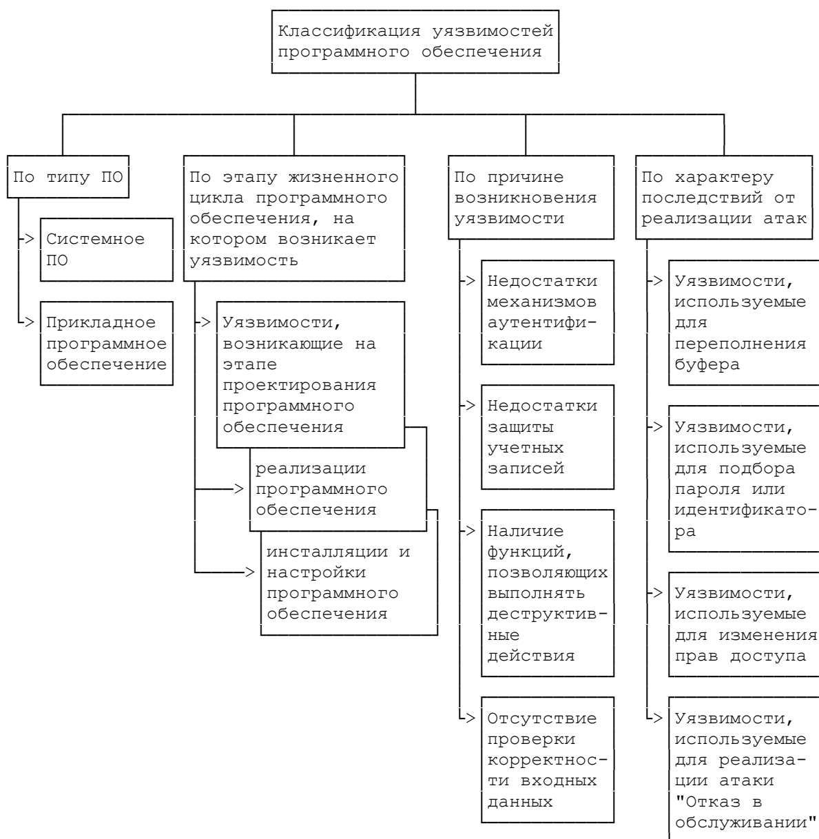
Рисунок 4. Классификация уязвимостей программного обеспечения
