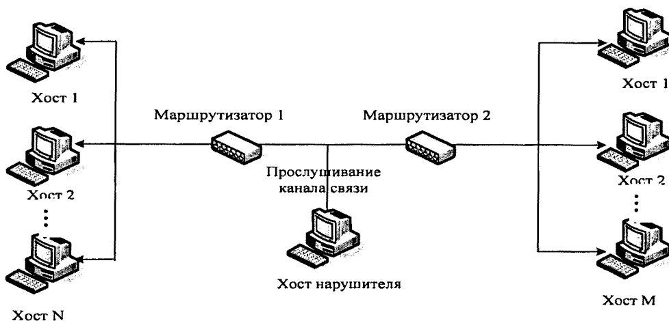
Рисунок 6. Схема реализации угрозы "Анализ сетевого трафика"
